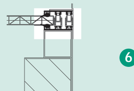
Detail 6 Beëindiging zijkant ter plaatse van opgaand werk. Over de hoeklijst kunnen loodketen aangebracht worden (zelfdragend systeem)
