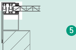
Detail 5 Beëindiging zijkant met kantlijst 3013 (zelfdragend systeem)
