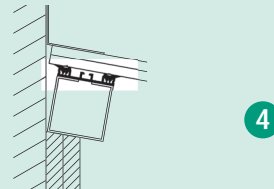
Detail 4 Doorsnede glaslijst 3198 ter plaatse van aansluiting muurzijde (zelfdragend systeem)
