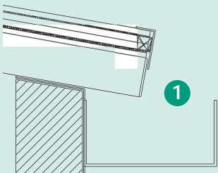
Detail 1 Aansluiting aan gootzijde ter plaatse van het roede-profiel (zelfdragend systeem)
