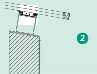
Detail 2 Doorsnede glaslijst 3198 ter plaatse van gootzijde (zelfdragend systeem)
